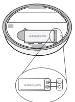
(2) Wymień na 1 baterię 6LR61 / 6F22.
